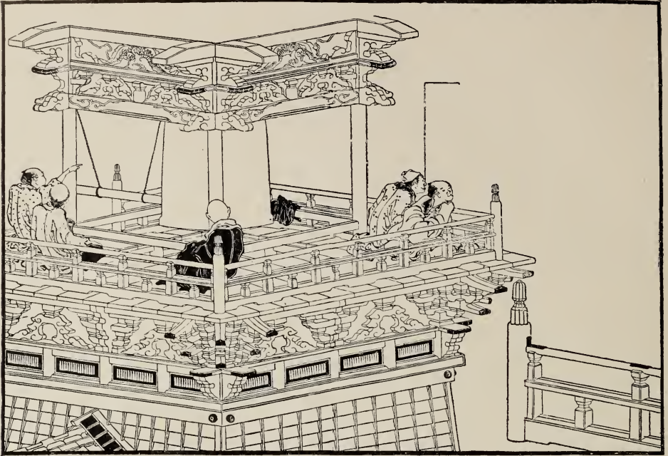
Abb. 94. Entwurf zum Mittelgeschoß des Glockenturms eines Tempels. Aus dem Shin hinagata. (Zu Seite 93.)
